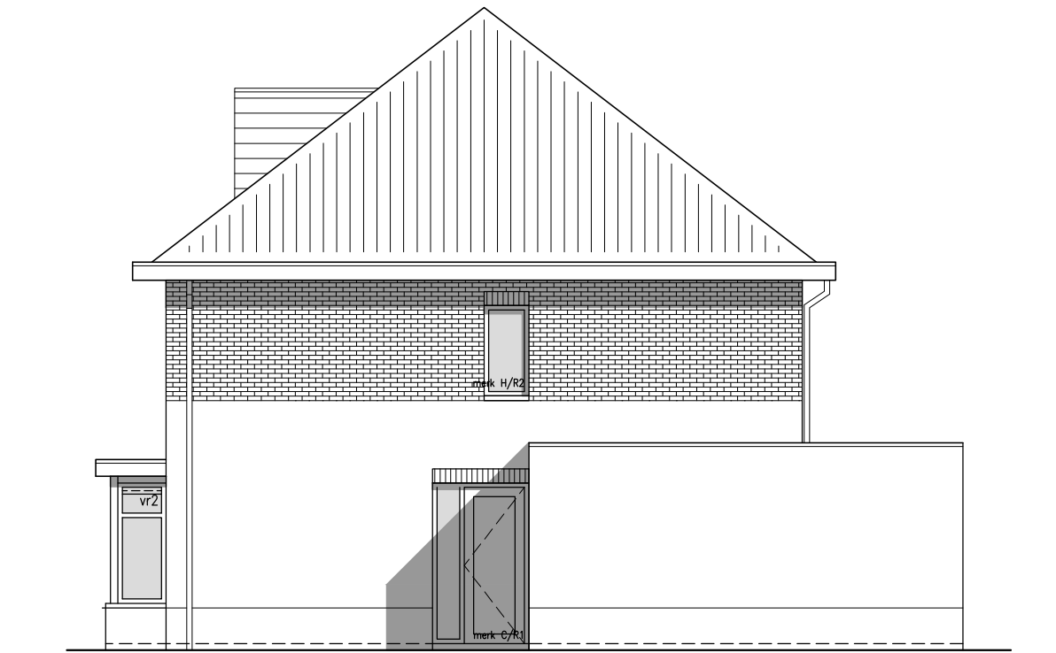
zijgevel rechts
